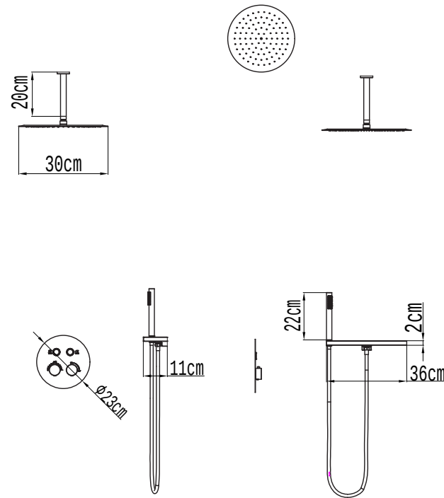
PRODUCT SIZE 产品尺寸
