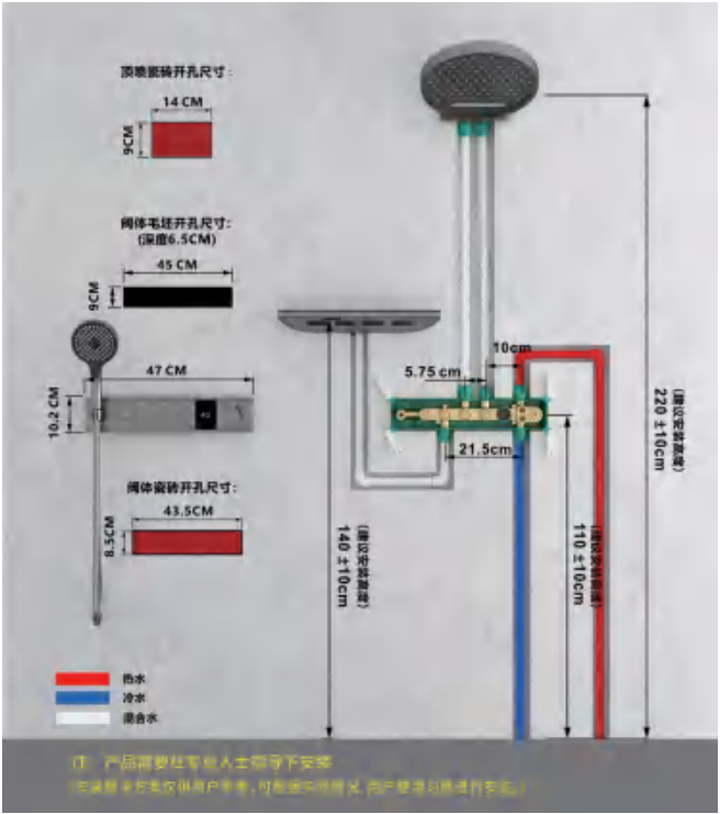
EMBEDDED PIPELINE 预埋管道
