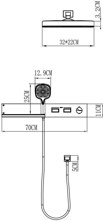
PRODUCT SIZE 产品尺寸
