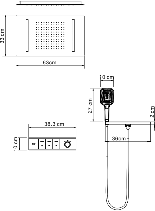
PRODUCT SIZE 产品尺寸
