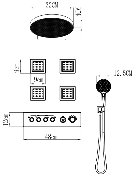
PRODUCT SIZE 产品尺寸
