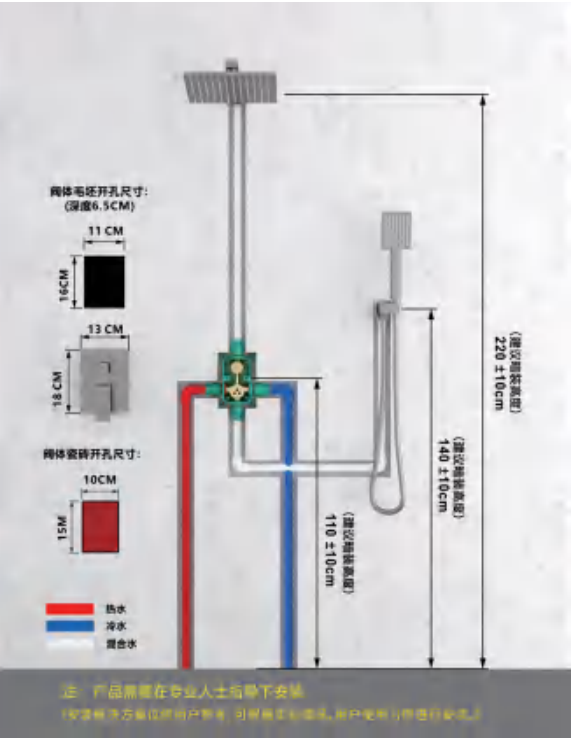
EMBEDDED PIPELINE 预埋管道
