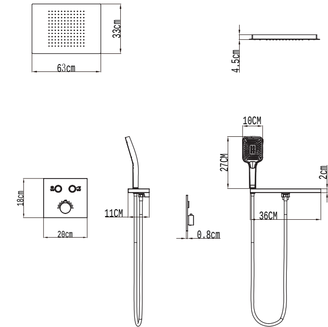
PRODUCT SIZE 产品尺寸
