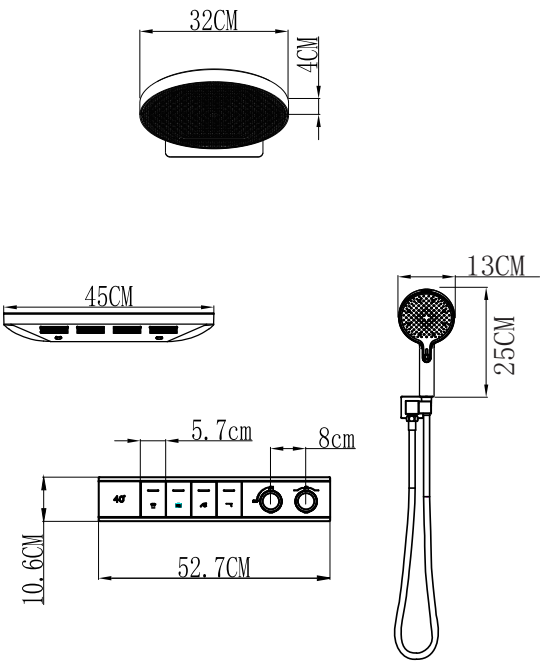
PRODUCT SIZE 产品尺寸
