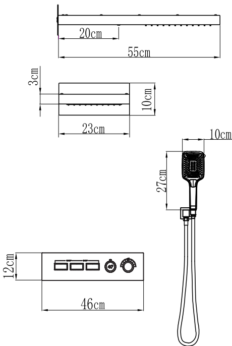
PRODUCT SIZE 产品尺寸
