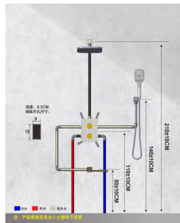
EMBEDDED PIPELINE 预埋管道
