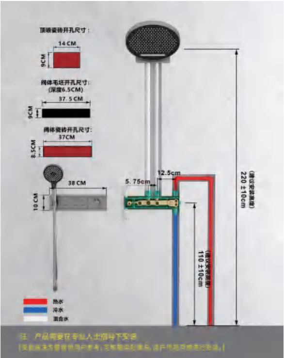
EMBEDDED PIPELINE 预埋管道
