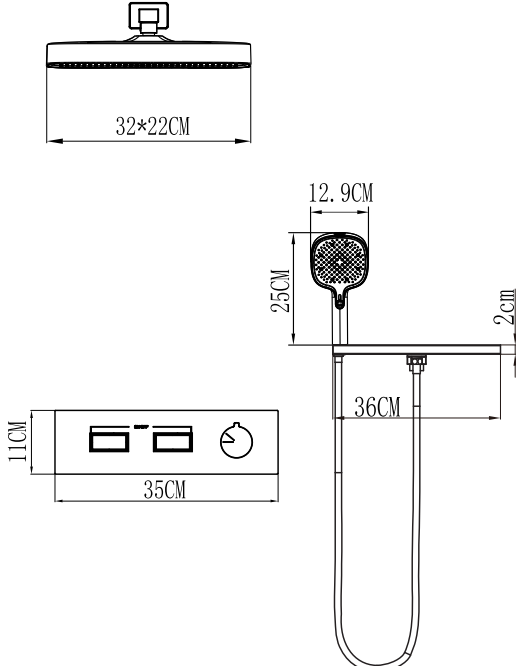
PRODUCT SIZE 产品尺寸
