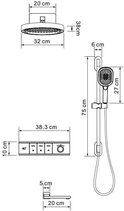
PRODUCT SIZE 产品尺寸
