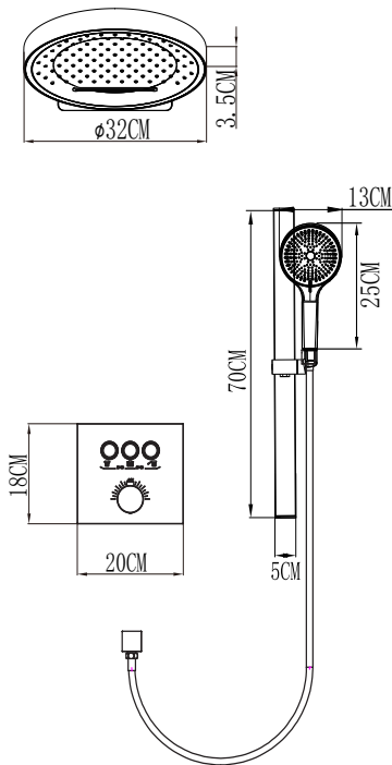
PRODUCT SIZE 产品尺寸
