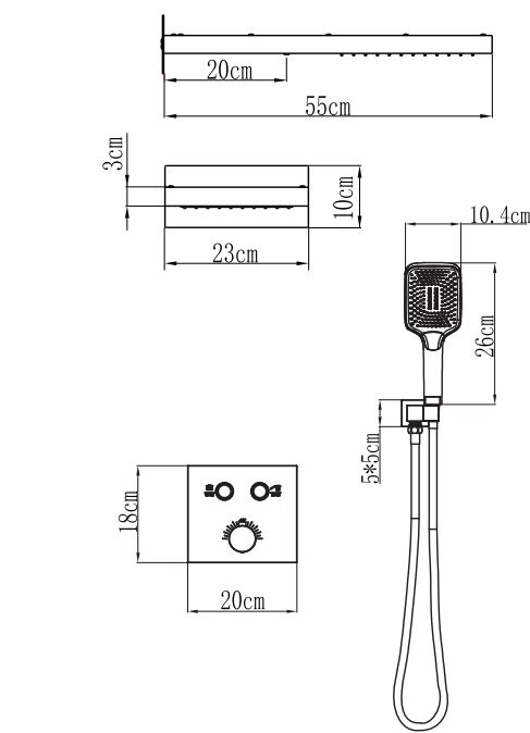
PRODUCT SIZE 产品尺寸
