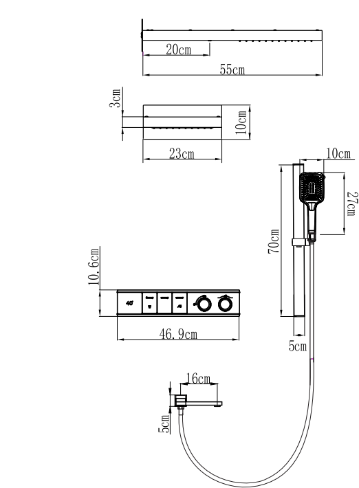
PRODUCT SIZE 产品尺寸
