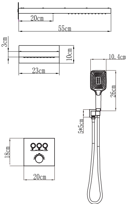
PRODUCT SIZE 产品尺寸
