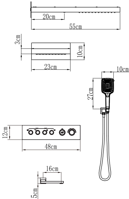
PRODUCT SIZE 产品尺寸
