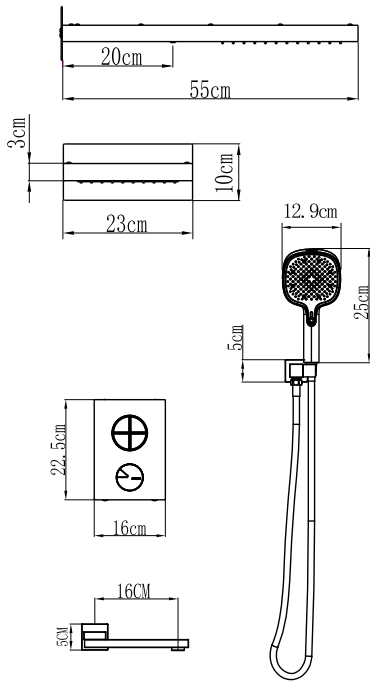
PRODUCT SIZE 产品尺寸
