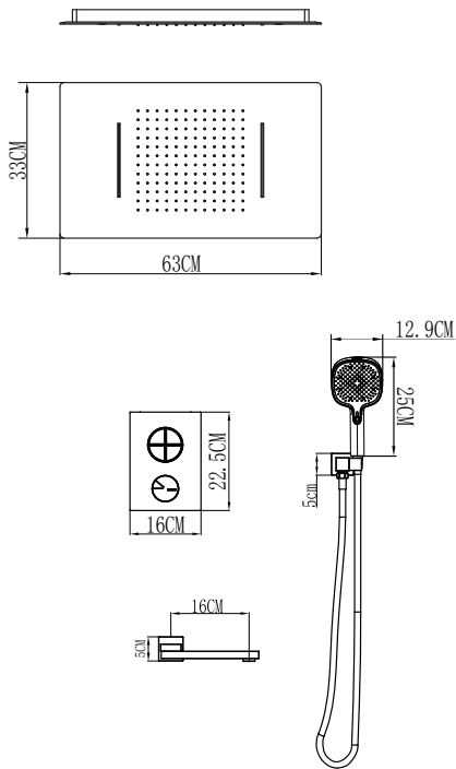
PRODUCT SIZE 产品尺寸
