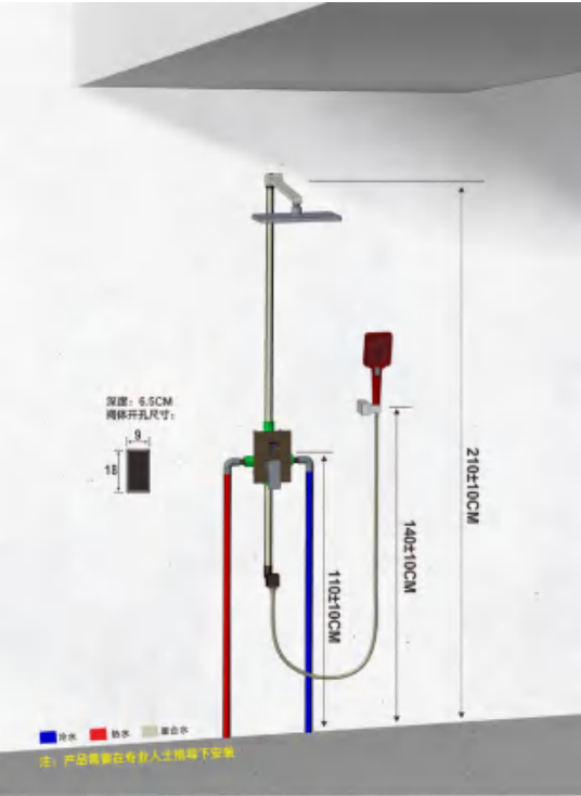
EMBEDDED PIPELINE 预埋管道
