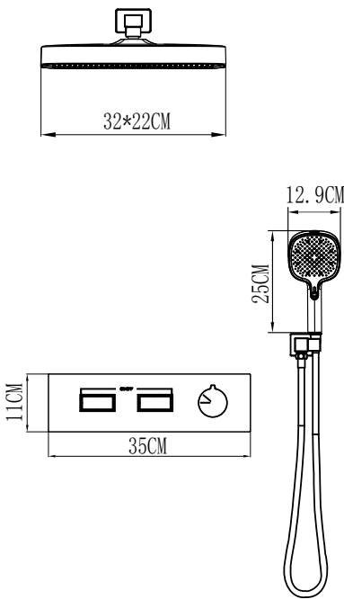
PRODUCT SIZE 产品尺寸
