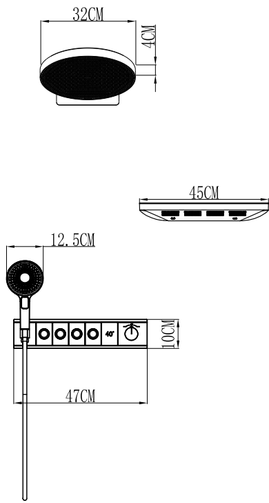
PRODUCT SIZE 产品尺寸
