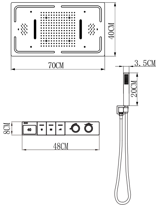
PRODUCT SIZE 产品尺寸
