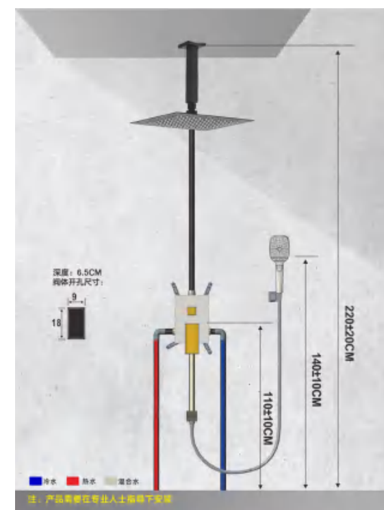
EMBEDDED PIPELINE 预埋管道
