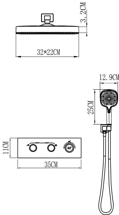
PRODUCT SIZE 产品尺寸
